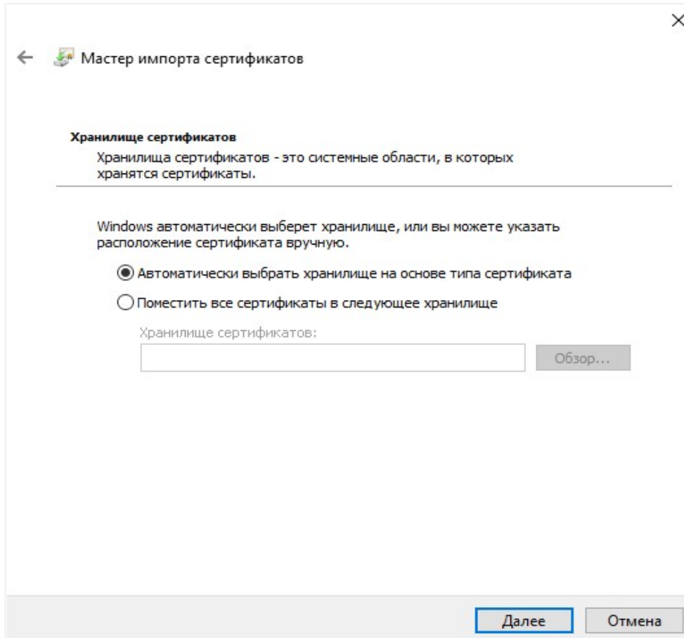
Рисунок 15 – Хранилище сертификатов
