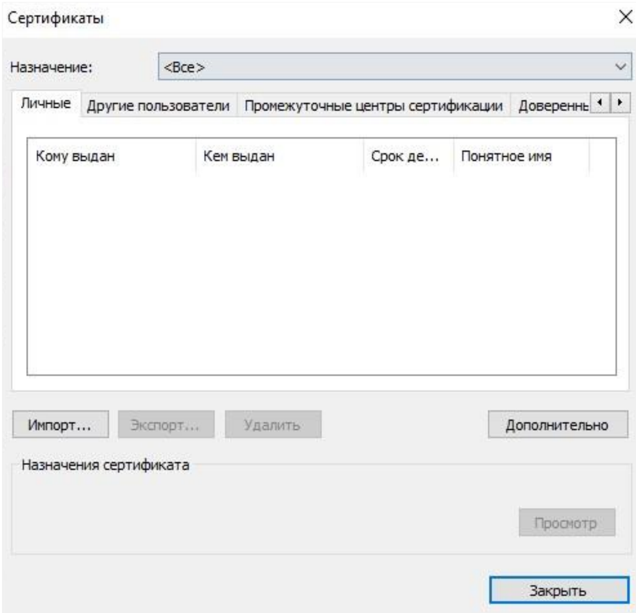
Рисунок 108 – Страница «Сертификаты»
