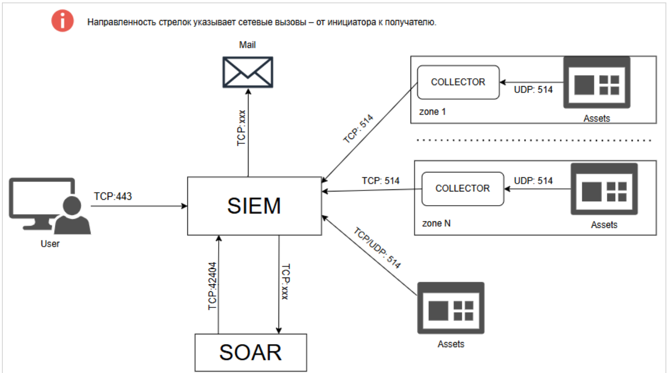
Рисунок 1 – Схема взаимодействия компонентов для версии NT SIEM
