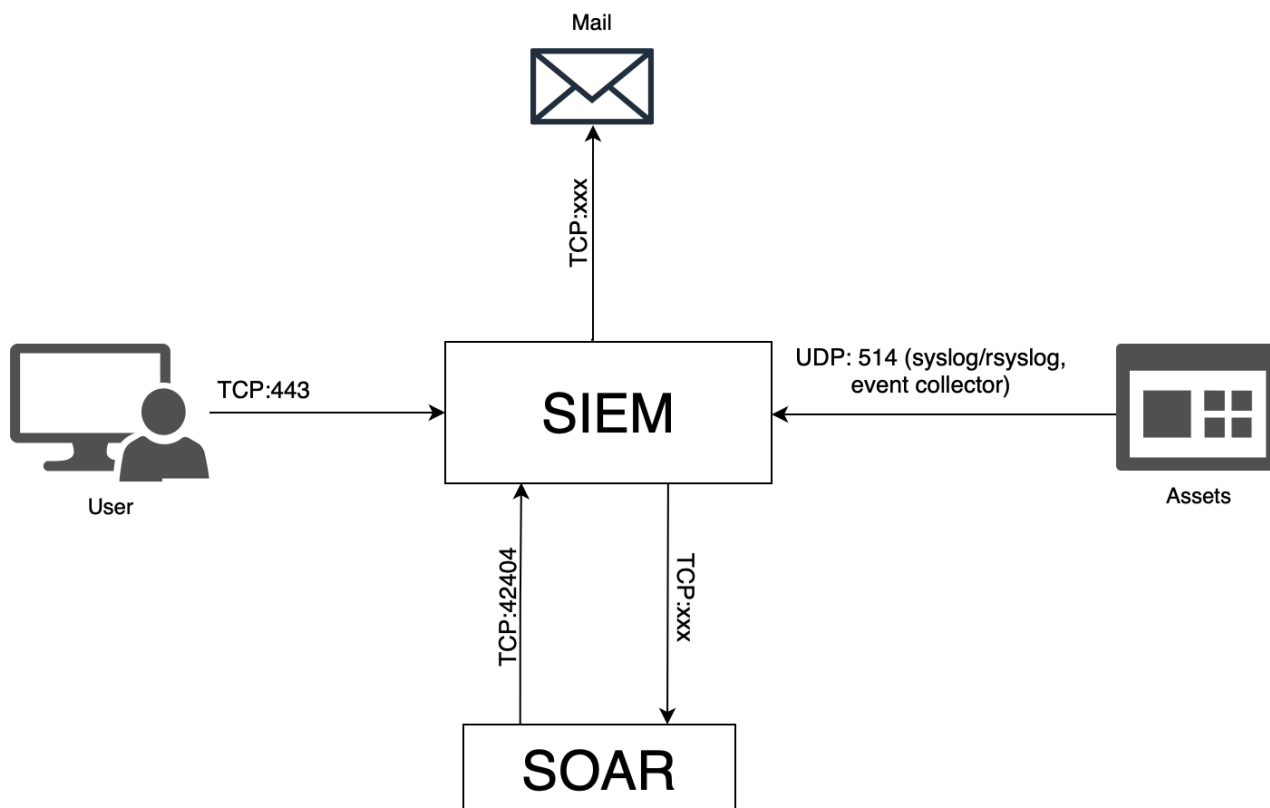
Рисунок 1 – Схема взаимодействия компонентов для версии NT SIEM v2.0.0
