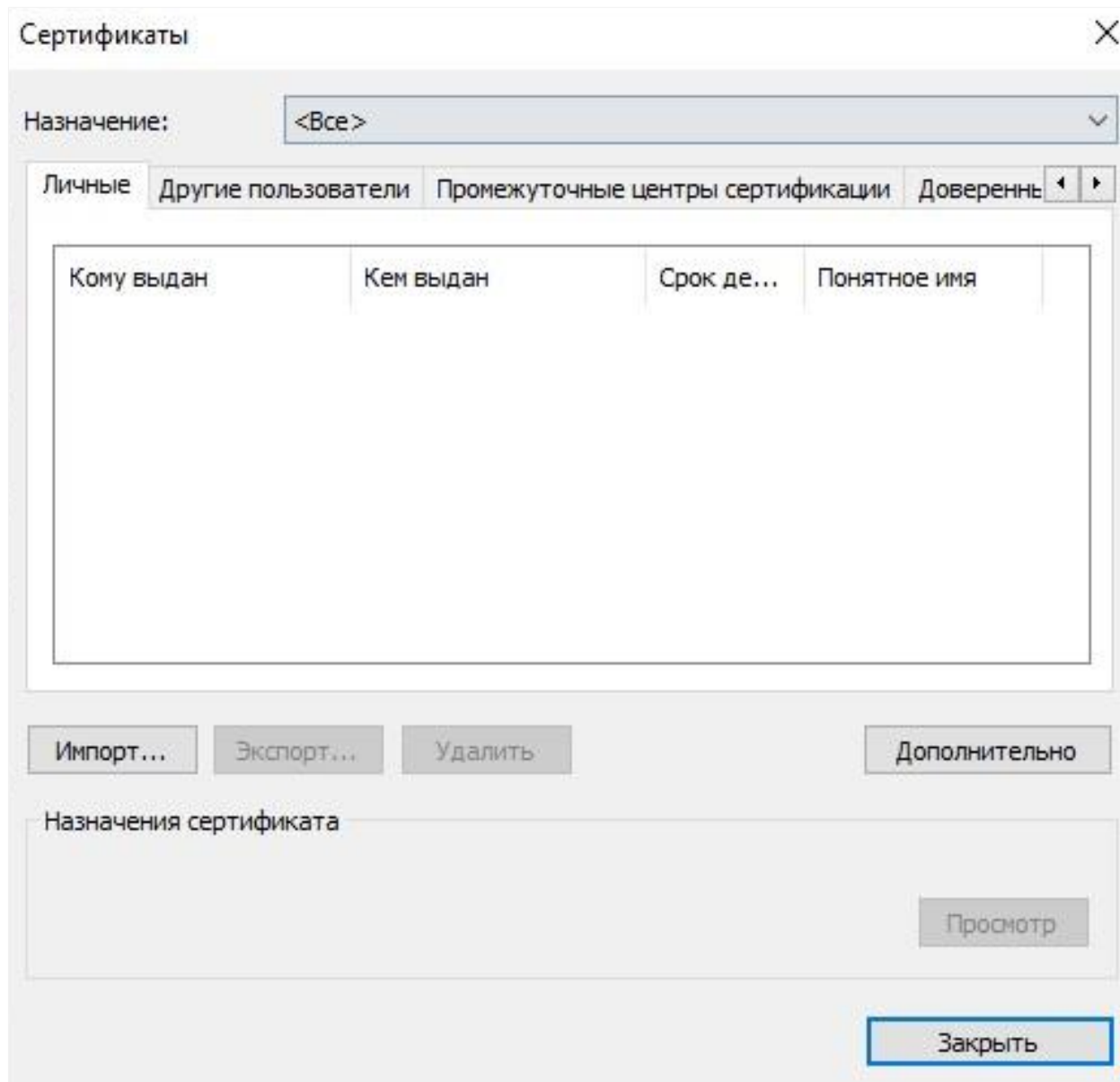
Рисунок 11 – Страница «Сертификаты»
