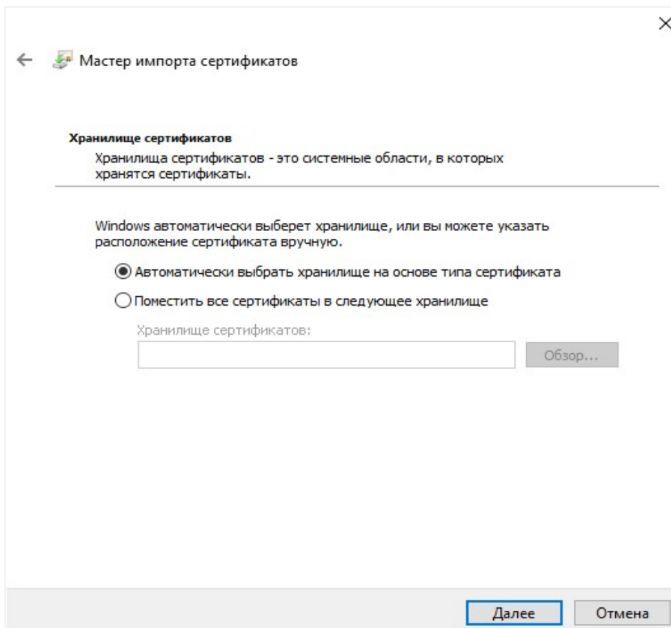
Рисунок 8 – Хранилище сертификатов
