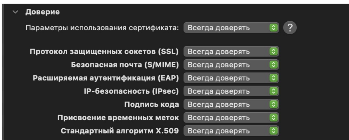
Рисунок 10 – Вкладка «Доверие» приложения «Связка ключей»
