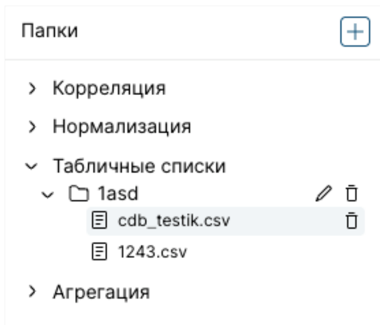
Рисунок 59 – Удаление файла
