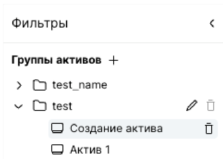
Рисунок 44 – Удаление актива
